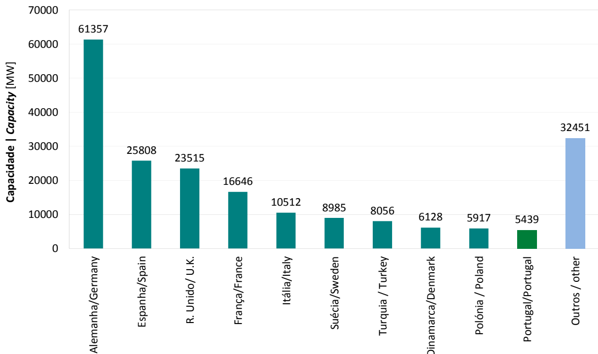
Figura 2: Capacidade geradora 2019 - Europa Figure 2: Installed capacity 2019 - Europe
