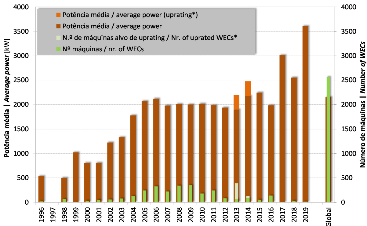
Figura 16: Número de aerogeradores e potência unitária média 1996-2019 Figure 16: Number of WECs and averagemean rated power 1996-2019
