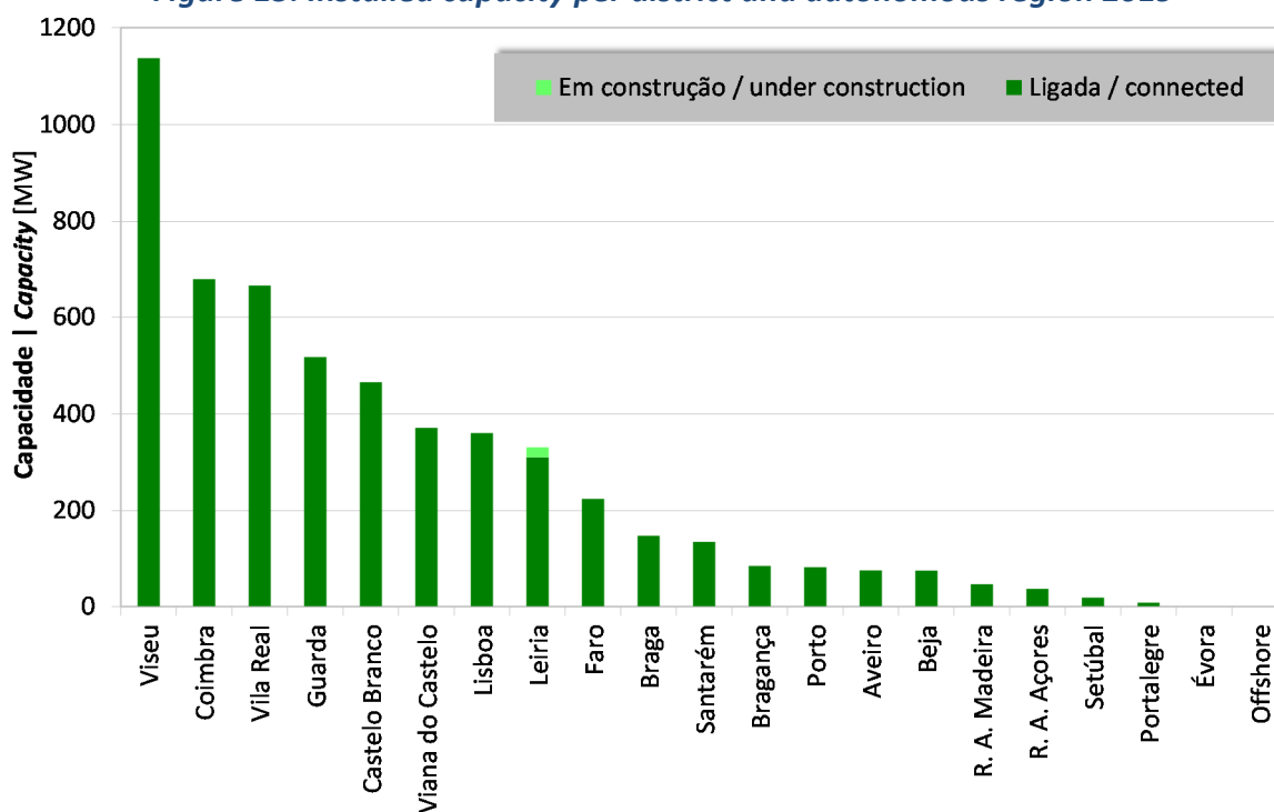
Figura 13: Potência Instalada por Distrito e Região Autónoma 2019 Figure 13: Installed capacity per district and autonomous region 2019
