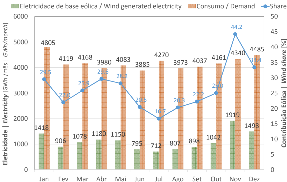
Figura 8: Geração eólica vs. Consumo de eletricidade 2019 Portugal Continental Figure 8: Wind generation vs. Electricity demand 2019 - Mainland Portugal
