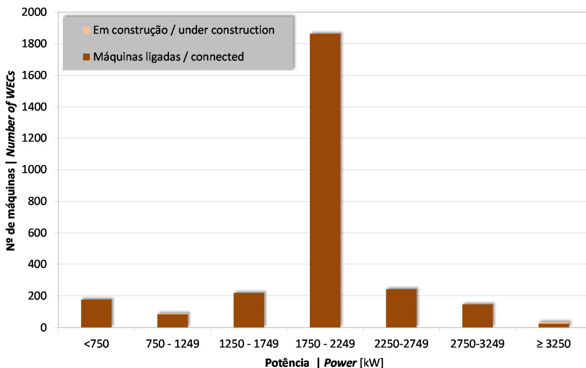
Figura 17: Número de aerogeradores por classe de potência 2019 Figure 17: Number of WECs by power class 2019
