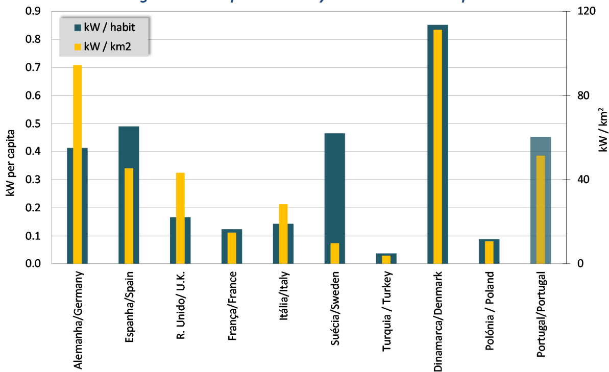
Figura 4: Índices de densidade 2019 - Europa Figure 4: Wind power density indexes 2019 - Europe
