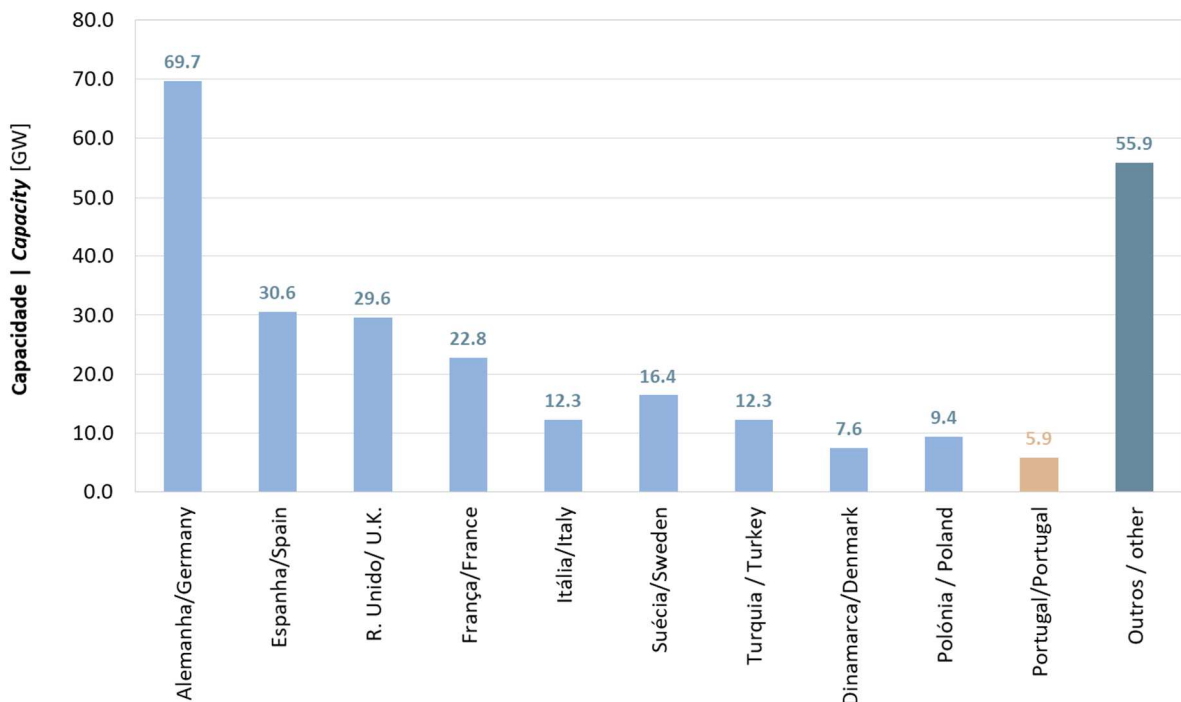
Figura 2: Capacidade geradora 2023 - Europa Figure 2: Installed capacity 2023 - Europe
