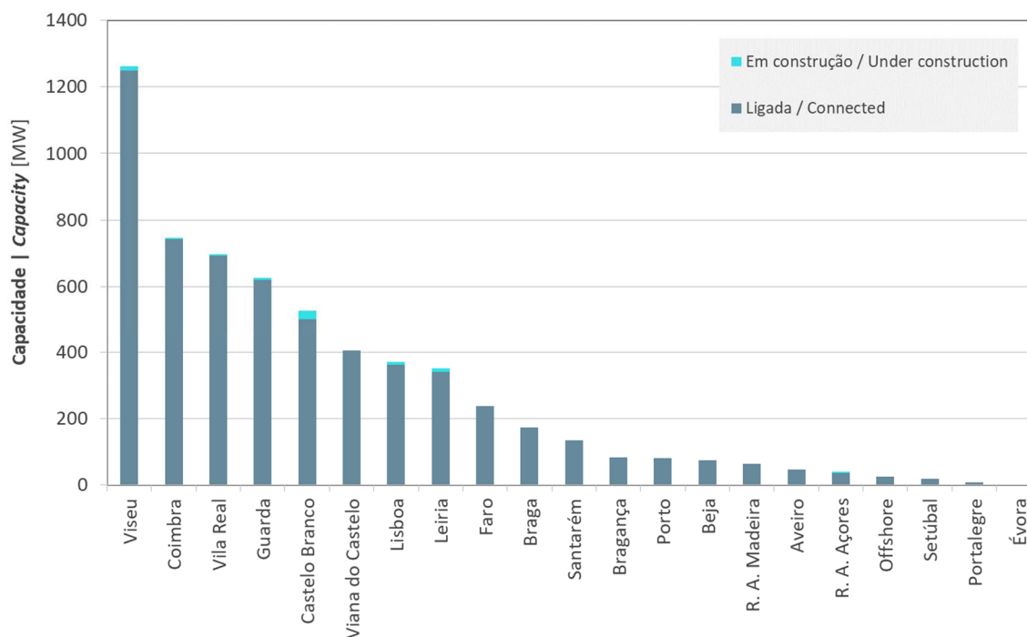
Figura 13: Potência Instalada por Distrito e Região Autónoma | 2023 Figure 13: Installed capacity per district and autonomous region | 2023
