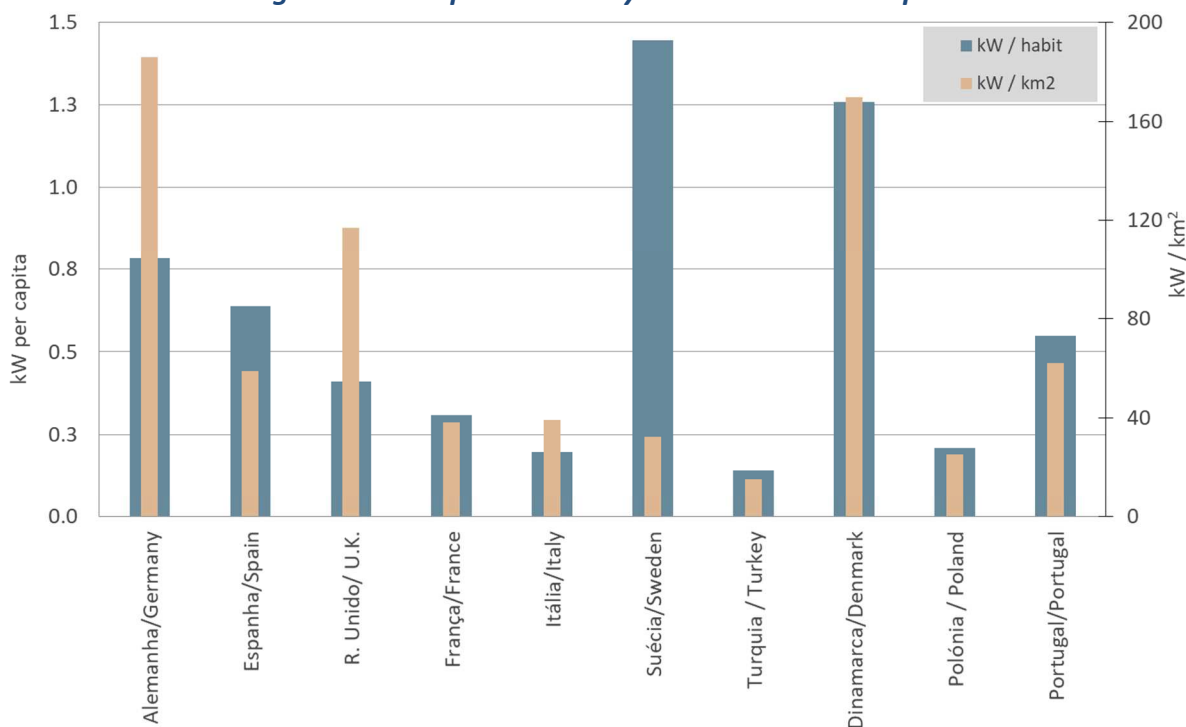
Figura 4: Índices de densidade 2023 - Europa Figure 4: Wind power density indexes 2023 - Europe
