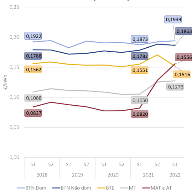
Figura 19 – Evolução dos preços por nível de tensão (sem IVA)
