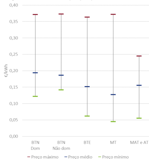
Figura 20 – Gama de preços por nível de tensão
